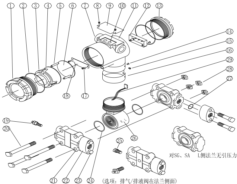
图 1.2 智能变送器整机结构
