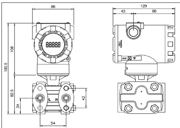
图 1.1 智能变送器外型尺寸（单位：mm）
