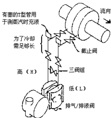
图 2.5 蒸汽介质连接示意图
