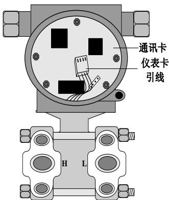
图 3.5 仪表卡与通讯卡连接
