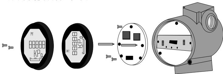
图 3.7 表头安装结构图
