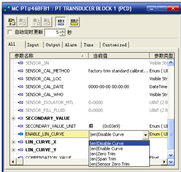
图6.3 ENABLE_LIN_CURVE 的配置
