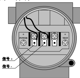
图 2.7 FF、PA 型智能变送器接线图
