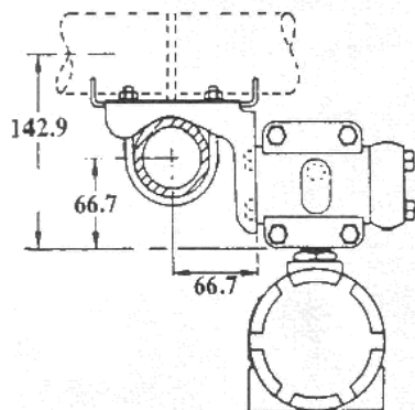
图 2.2 弯支架管装
