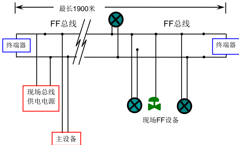
图6.2 FF 总线连接
