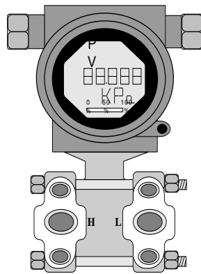
图 3.6 整机图
